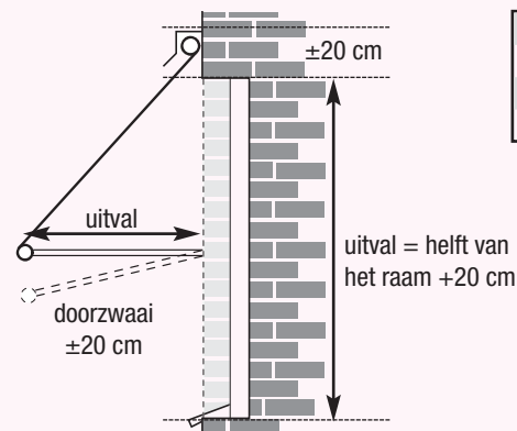
vaste arm
